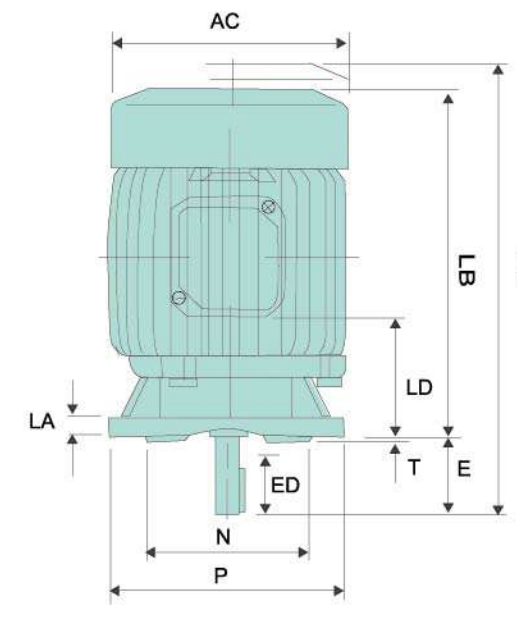
● 外型尺寸圖
